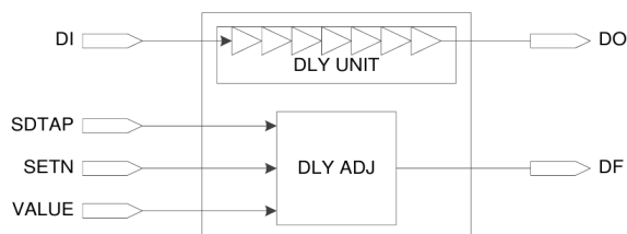
图 2-8 IODELAY 示意图
