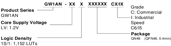
图 4-1 GW1AN-1S & 1 器件命名方法示例-Production
