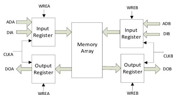
读写时钟模式
