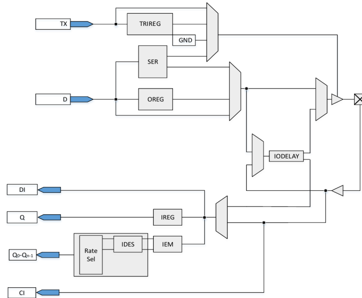
图 2-7 I/O 逻辑输入输出示意图
