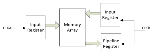
单端口时钟模式
