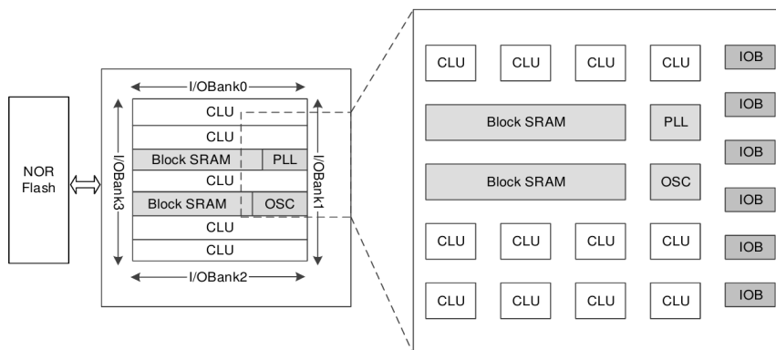
图 2-2 GW1AN-1 器件结构示意图
