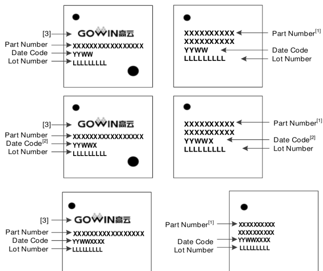
图 4-2 器件封装标识示例
