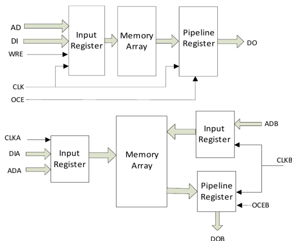
图 2-10 单端口、伪双端口及双端口模式下的流水线模式
