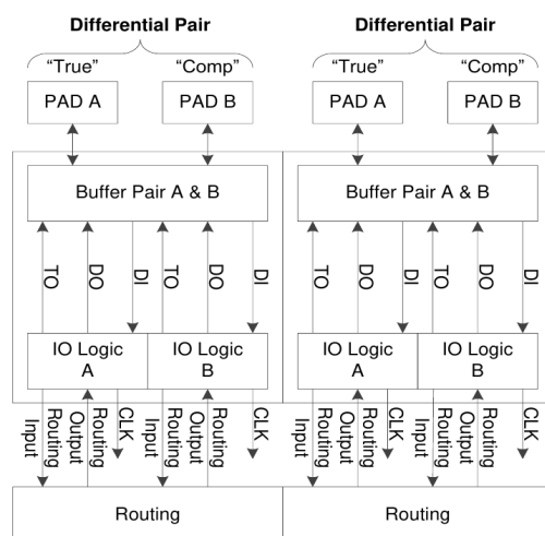
图 2-4 IOB 结构示意图
