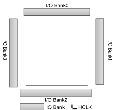
图 2-15 GW1AN-1 HCLK 示意图
