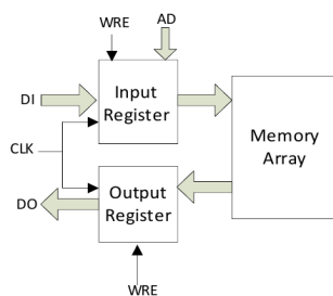
图 2-13 单端口时钟模式
