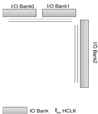
图 2-14 GW1AN-1S HCLK 示意图
