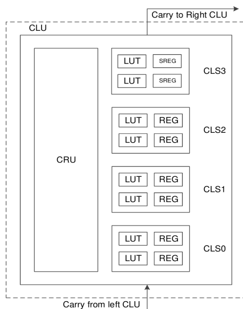
图 2-3 CLU 结构示意图
