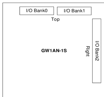
图 2-5 GW1AN-1S I/O Bank 分布示意图
