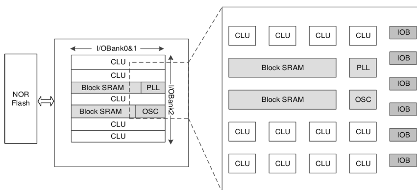
图 2-1 GW1AN-1S 器件结构示意图
