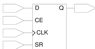
图 2-9 I/O 寄存器示意图
